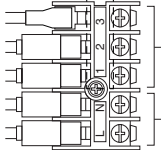
Stroomkabel Verbindingskabel tussen buitenunit en binnenunit
