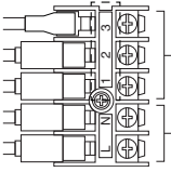
Güç beslemesi (dış ve iç ünite kablosu arasındaki bağlantı kablosu)
