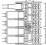
Καλώδιο σύνδεσης ηλεκτρικής παροχής και εσωτερικής μονάδας
