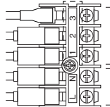
Câble d'alimentation électrique
