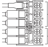
Захранващ кабел между външно и вътрешно тяло
