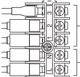
Stromversorgungskabel (zwischen Außen- und Inneneinheit)
