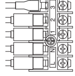
Câble de raccordement entre l'unité intérieure et extérieure
