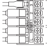
Свързващ кабел между външно и вътрешно тяло
