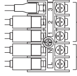
Stroomkabel Verbindingkabel tussen buitenunit en binnenunit
